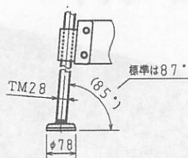
アウトリガー (S = 1 : 10)
